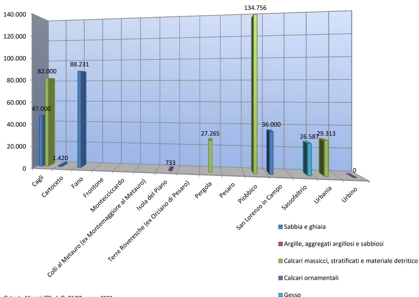
Volumi utili scavati nel 2021 in Provincia di Pesaro e Urbino
